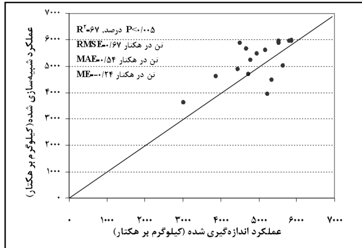
شکل ۲- نتایج صحت سنجی مدل AquaCrop برای گندم در سال زراعی ۸۳-۱۳۸۲ در شبکه آبیاری آبشار
