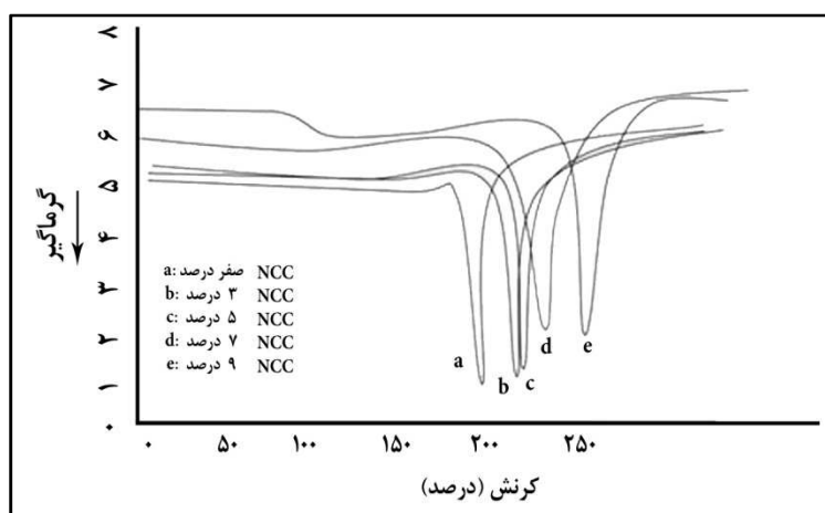
شکل ۶- منحنی‌های گرماسنجی پویایی تفاضلی فیلم‌های نانوکامپوزیت نشاسته، حاوی درصدهای مختلف نانوبلور سلولز
