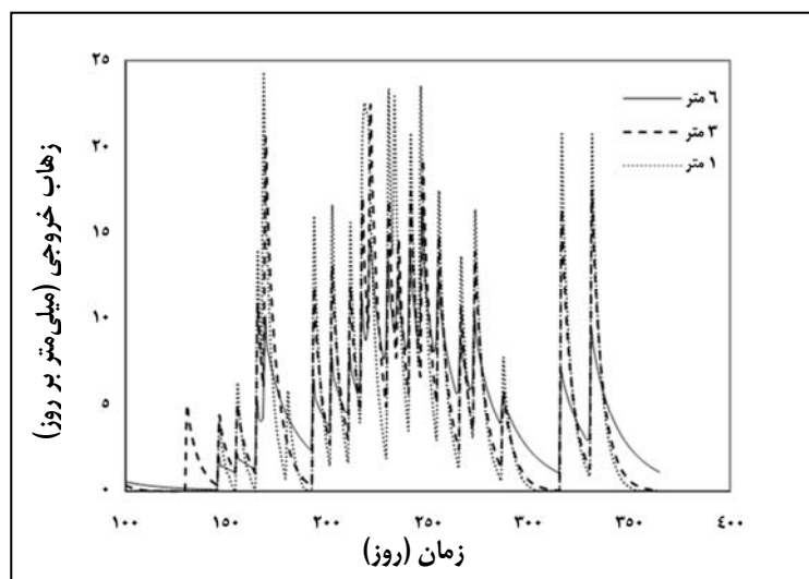
شکل ۴- تغییرات میزان زه‌اب خروجی در عمق‌های مختلف زهکش
