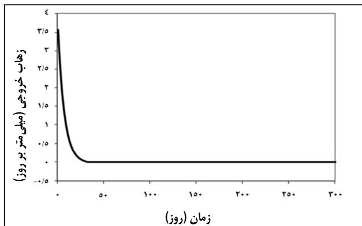
شکل ۳- تغییرات زه‌اب خروجی تحت شرایط حدی
