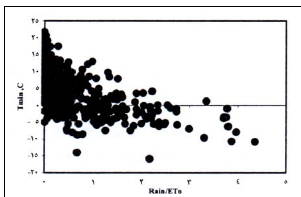
شکل شماره ۲- نمودار T_{\min} در مقابل \text{Rain}/\text{ET}_0 ، بررسی سالانه، مشهد
