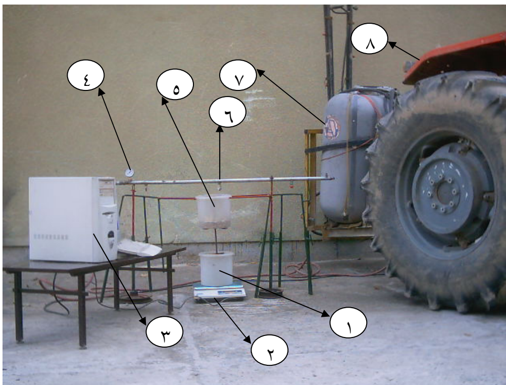
شکل شماره ۱- مکانیزم مورد استفاده برای اجرای آزمایش: ۱- ظرف جمع‌آوری زه آب ۲- ترازوی دیجیتال ۳- سیستم ثبت داده‌ها ۴- فشارسنج ۵- ظرف حاوی نمونه کاه ۶- افشانک ۷- سیستم پاشش و ۸- تراکتور
