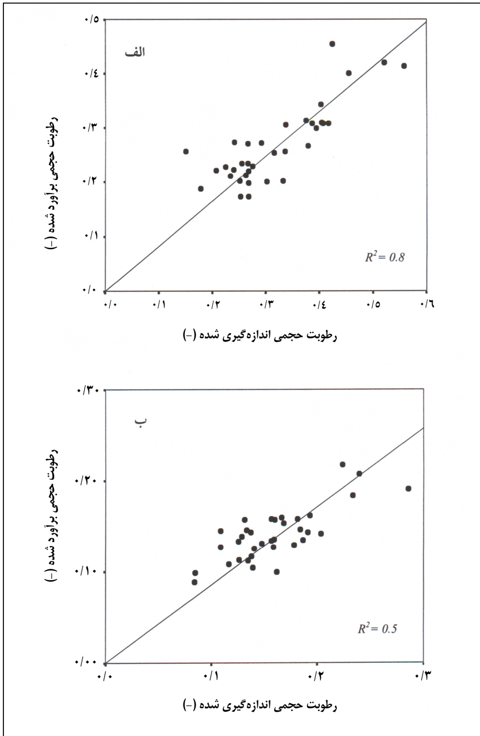
شکل شماره ۱- همبستگی رطوبت‌های اندازه‌گیری و برآورد شده با استفاده از توابع انتقالی نوع اول: (الف) برای پتانسیل ماتریک ۱۰- کیلوپاسکال، (ب) ۱۵۰۰- کیلوپاسکال
