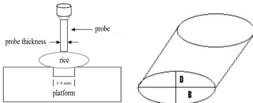
شکل ۲- طرح‌واره آزمون سه نقطه‌ای خمشی (چپ) و دانه برنج (راست).
