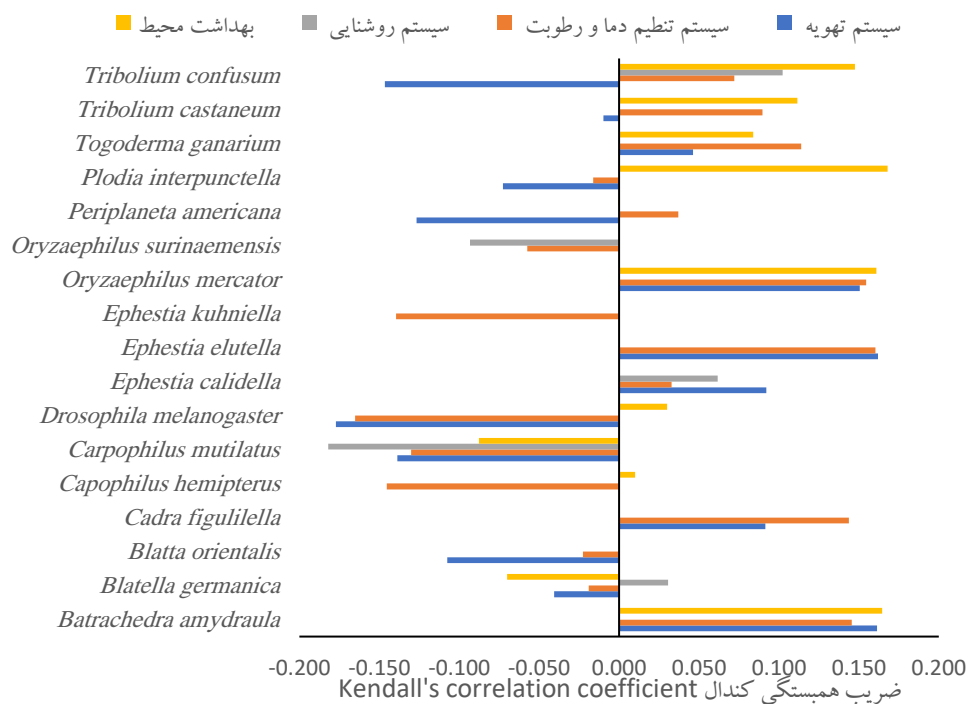
شکل ۳- ضرایب همبستگی کندال میان شاخص‌های استاندارد محیطی با جمعیت حشرات آفات انباری در شش استان خرم‌خیز ایران Figure 3- Kendall's correlation coefficients between standard environmental indicators and insect populations of storage pests in six date-producing provinces of Iran
