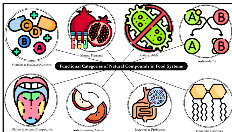
شکل ۳- طبقه‌بندی کارکردی ترکیبات طبیعی در سامانه‌های غذایی
